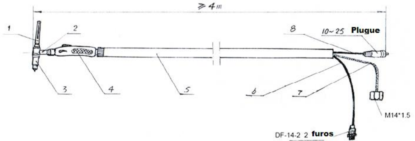
Figura: Vista explodida da tocha tig
